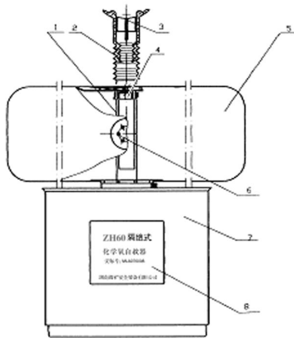
ZH30 (D) 隔绝式化学氧自救器结构原理图
